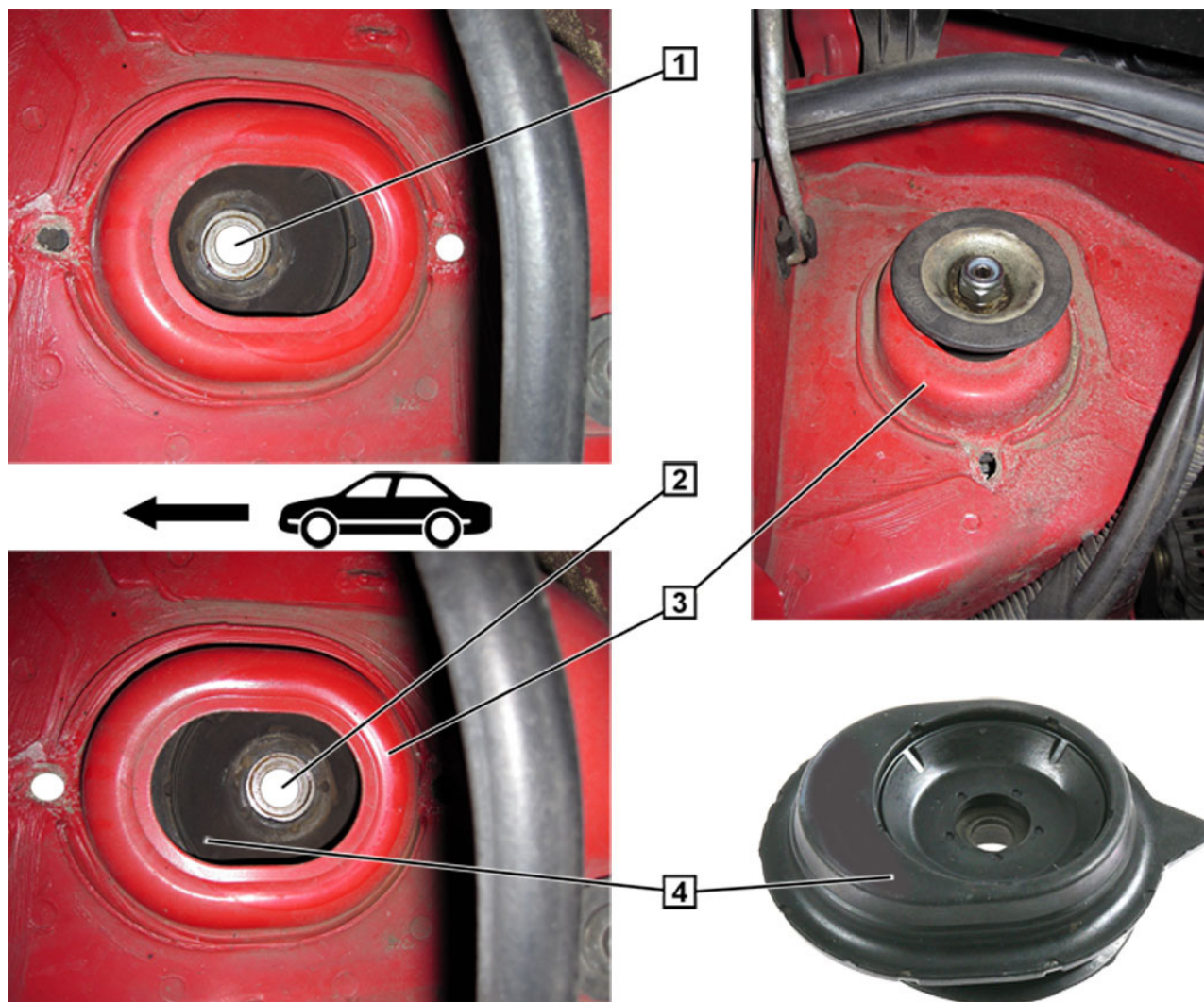
Sl. 1: Osloni ležaj opružne poluge na različitim mjestima ugradnje
