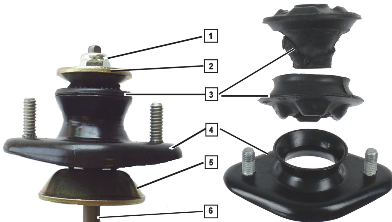
Sl. 1: netaknuti osloni ležaj opružne poluge s dijelovima za ugradnju
