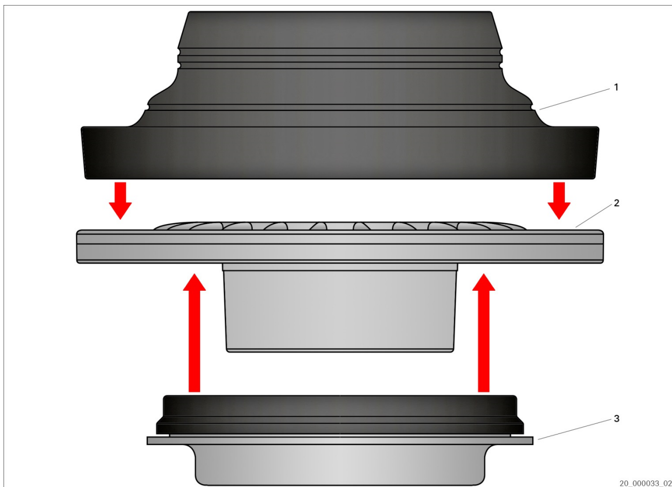
Fig. 1: assemblaggio del cuscinetto di supporto per montante telescopico (esempio)
