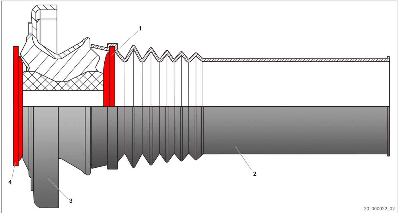
Fig. 1: cuscinetto di supporto per montante telescopico con kit di servizio
