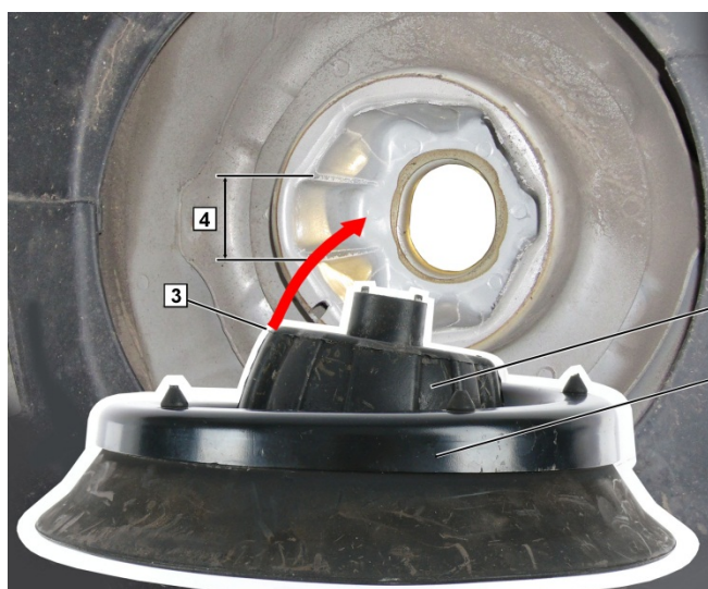
Εικ. 2: Θόλος γόνατου ανάρτησης
