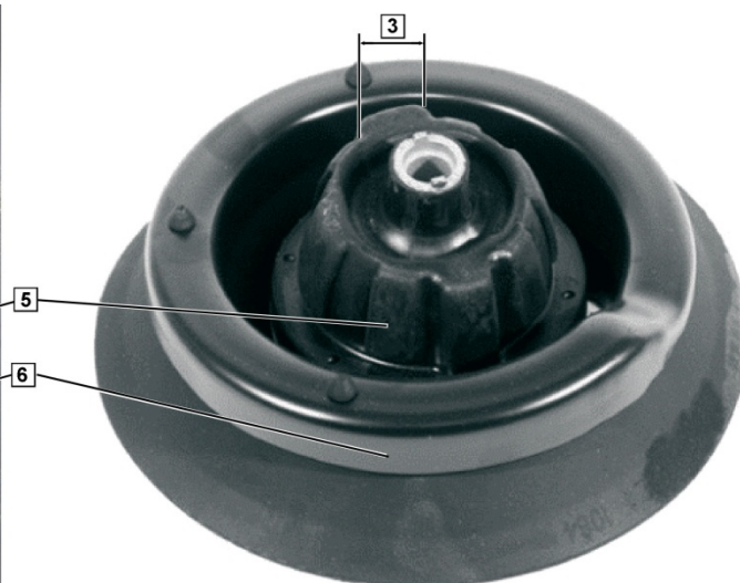
Εικ. 3: Έδρανο γόνατου ανάρτησης
