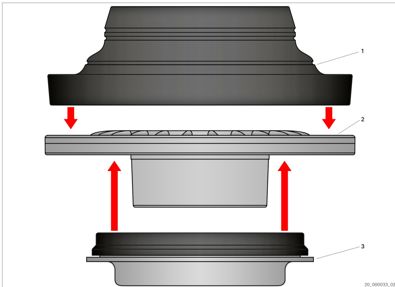
Фиг. 1: Сглобяване на опорния лагер на стойката на амортисьора (пример)
