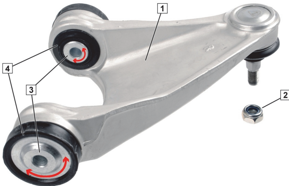
1. ábra: Keresztlengőkar
