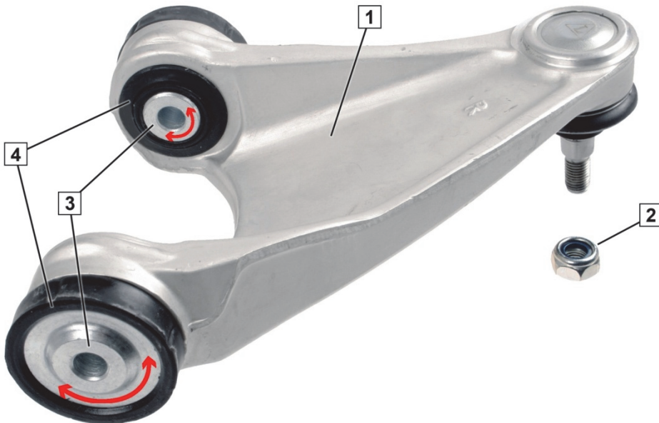
Slika 1: Poprečna obrtna poluga
