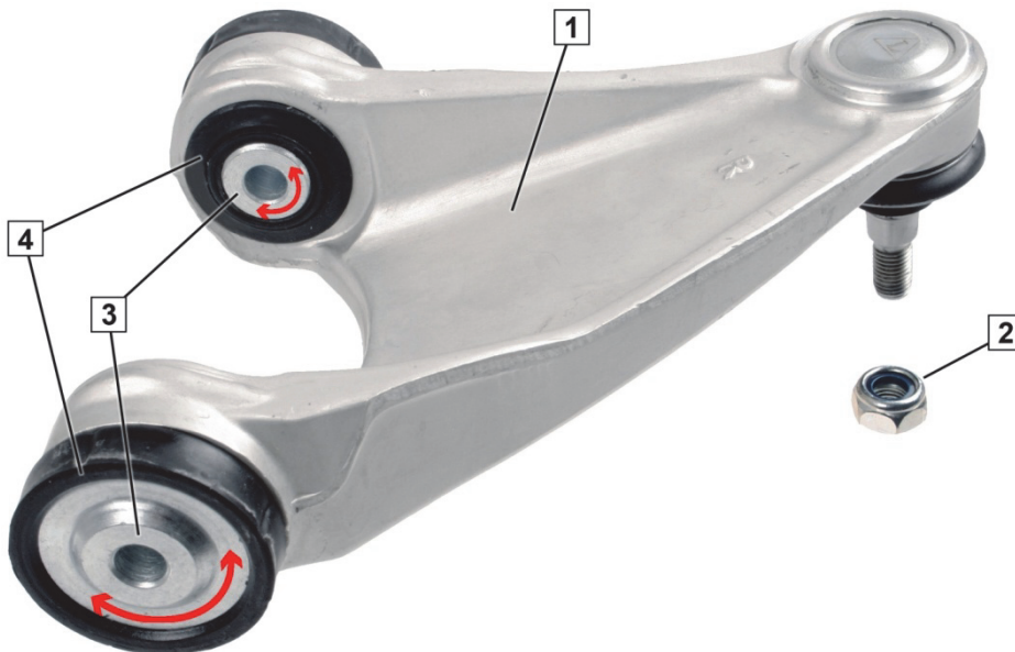
Рис. 1: Поперечный рычаг подвески
