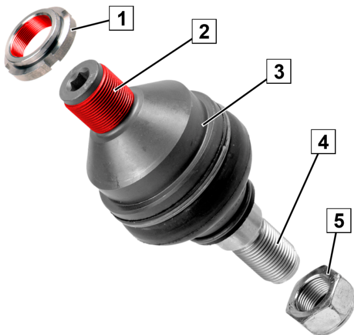
Fig. 1: Suspensão articulada
