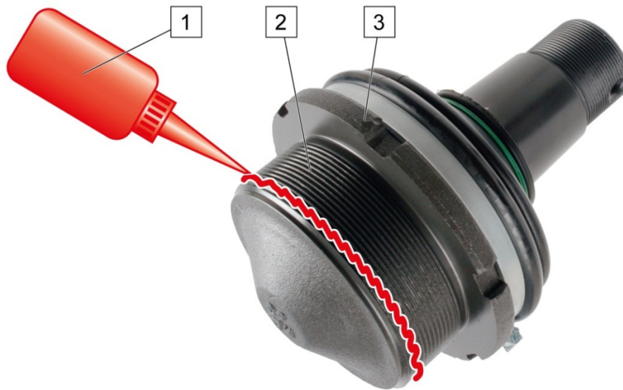
Εικ. 1: Άρθρωση ανάρτησης, μέσο ασφάλισης σπειρώματος
