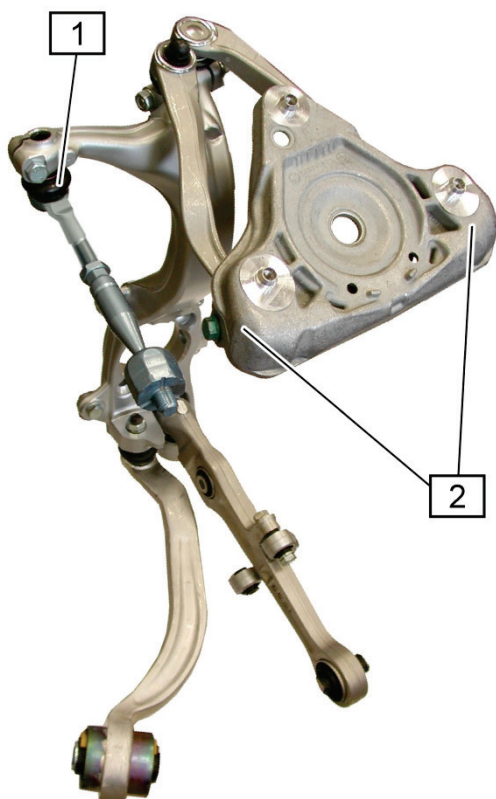
Fig. 1: Essieu avant Audi S-Line châssis
