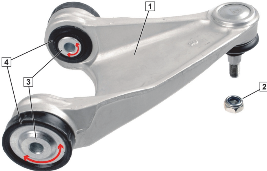
Fig. 1 : Bras oscillant transversal
