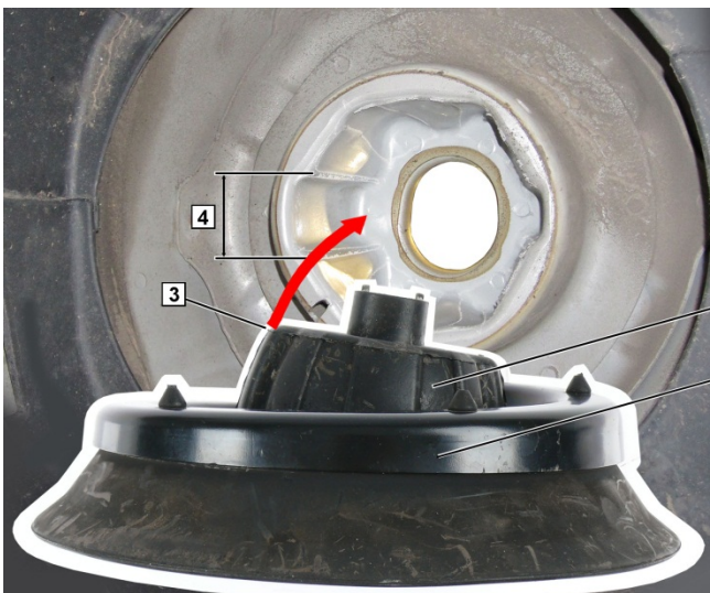
Fig. 2: cúpula del puntal de suspensión
