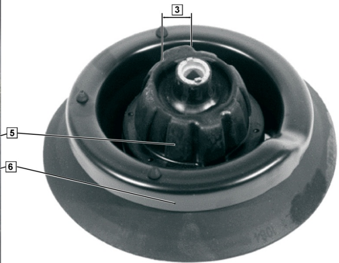
Fig. 3: soporte del puntal de suspensión
