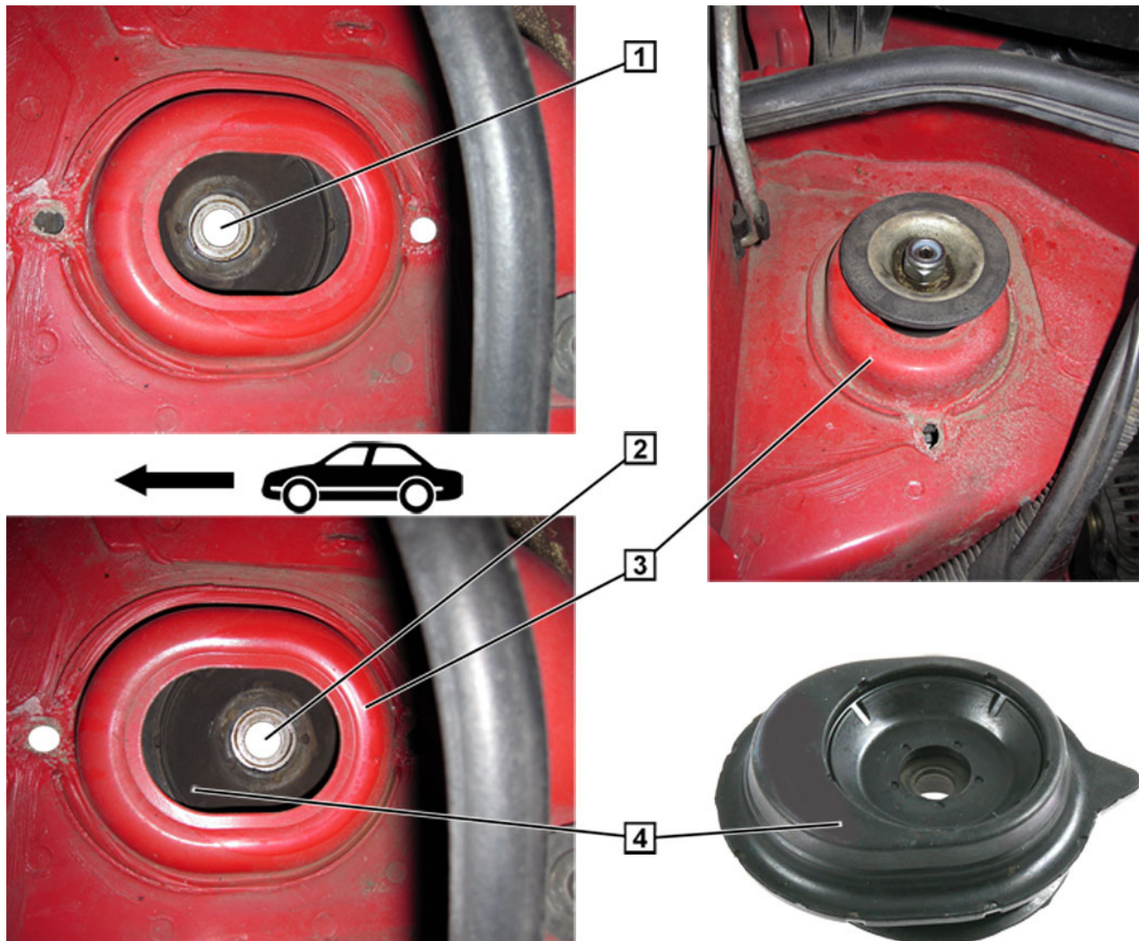
Fig. 1: Apoio superior do amortecedor em diferentes posições de montagem
