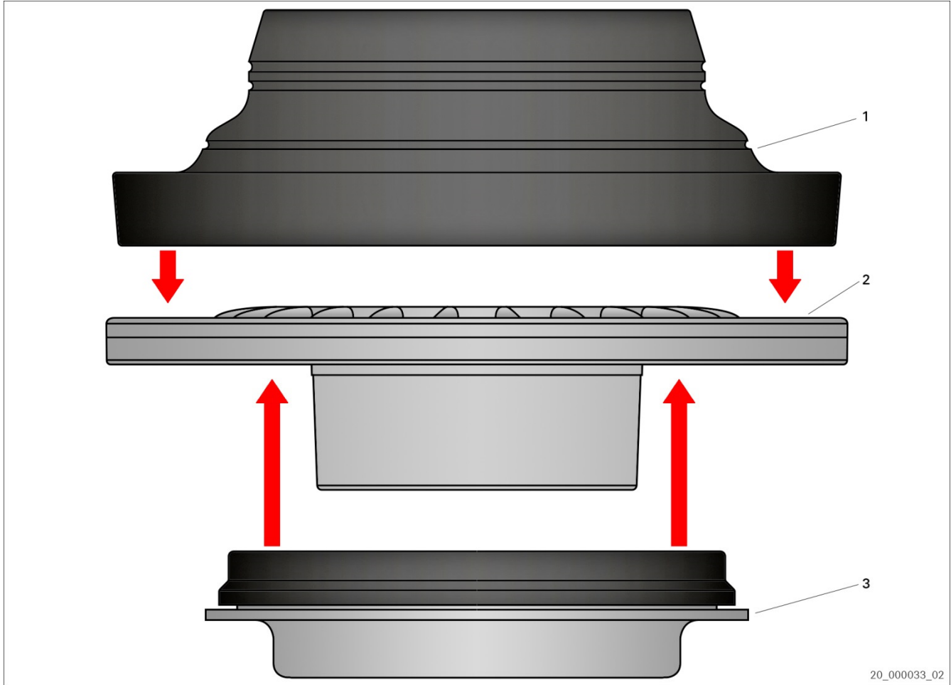
Şekil 1: Amortisör kule takozunun birleştirilmesi (örnek)
