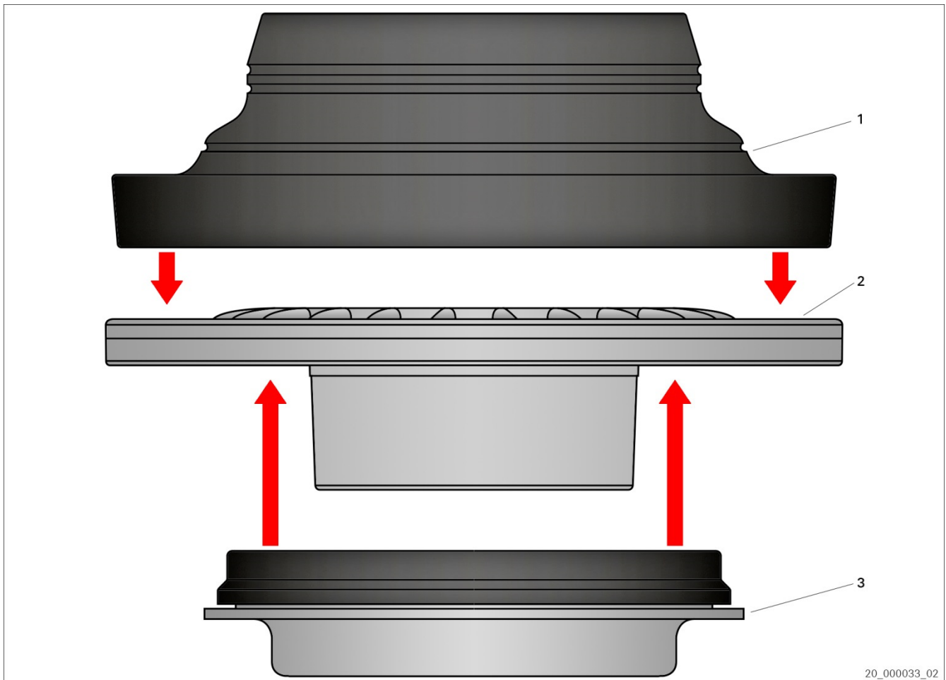
Obr. 1: Montáž opěrného ložiska pružící jednotky (příklad)
