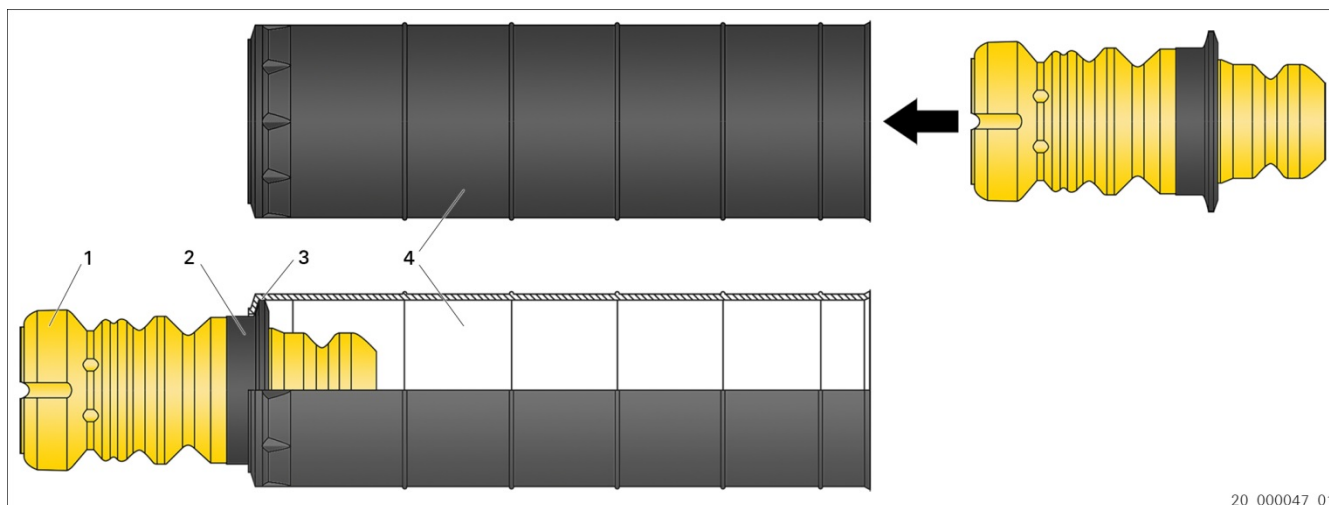
Sl. 1: Montaža kompleta za servisiranje (primer)
