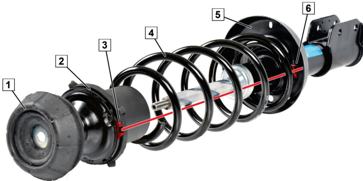
Afb. 1: Veerpootsteunlager correct geplaatst
