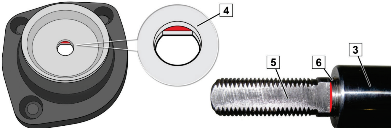
Afb. 1: Veerpootsteunlager en schokdemper achteras (10/2006 →)
