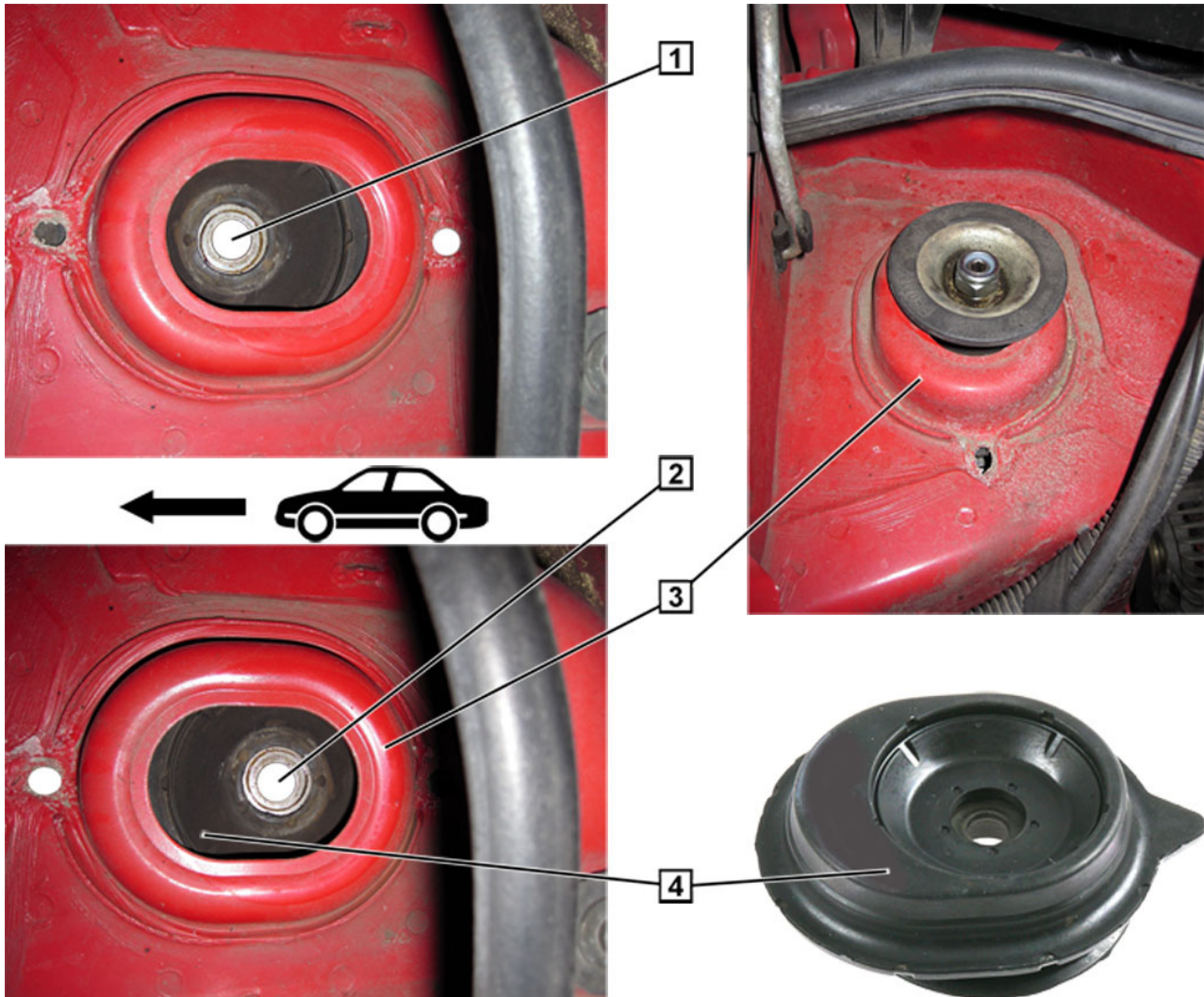
Fig. 1: Cuscinetti di supporto per montante telescopico in diverse posizioni di montaggio
