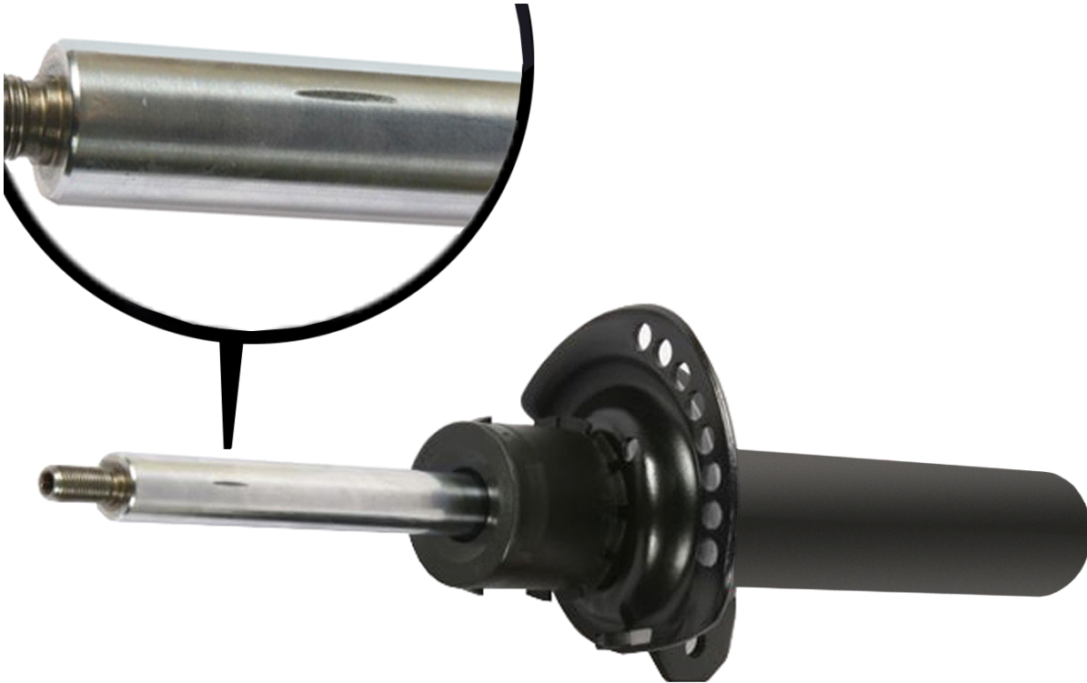
Kuva 1: Kiertokanki uralla
