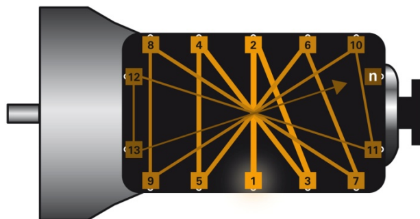
Obr. 1: Schematické zobrazenie poradia naskrutkovania
